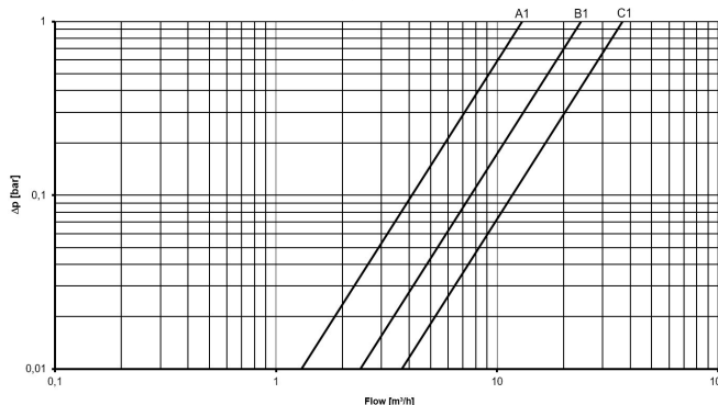
\Delta p flowIQ® 2200 & 3200 (KWM3231) Kompozit mérőtest
