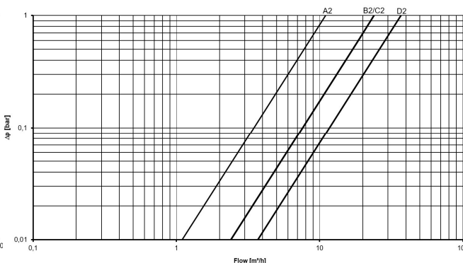
\Delta p flowIQ® 2200 & 3200 (KWM3231) Rozsdamentes acél mérőtest
