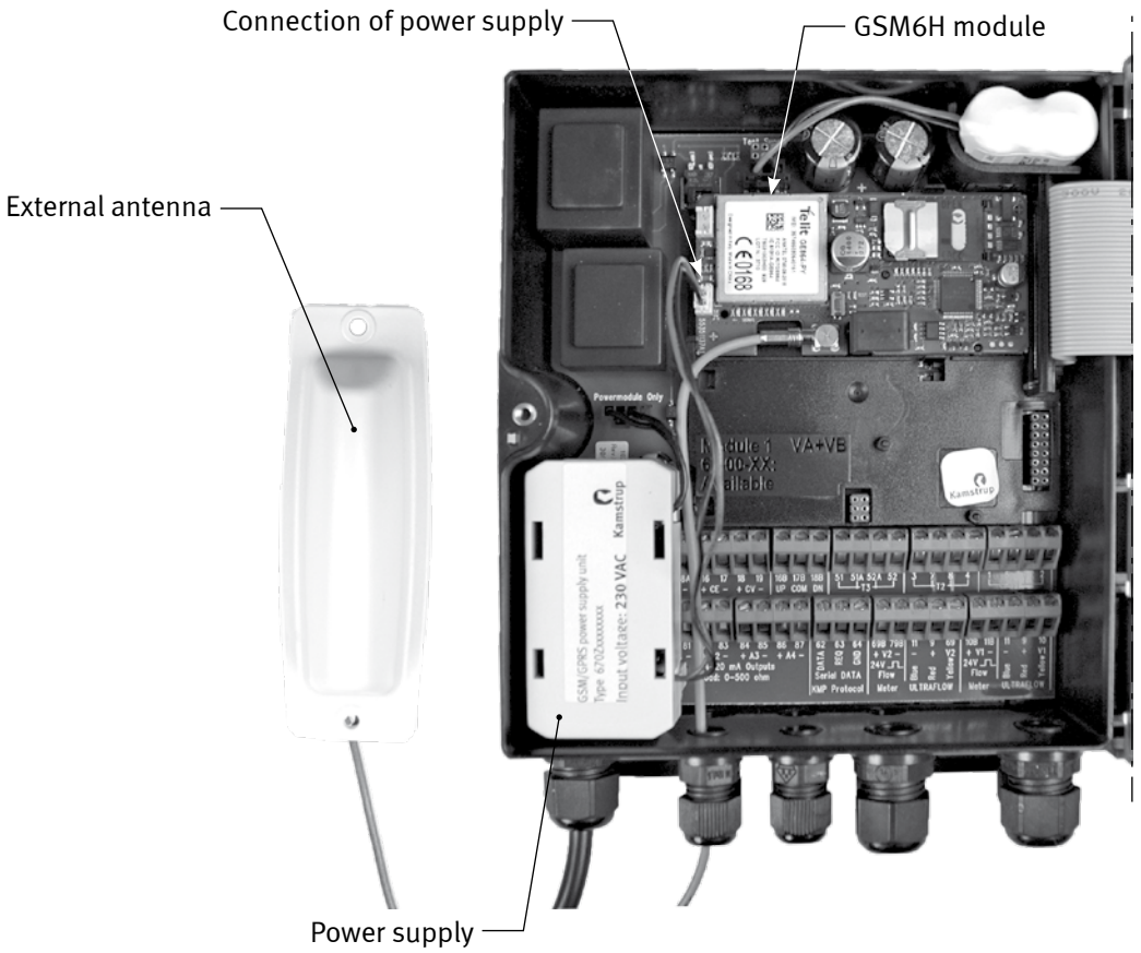
Fig. 3 – MULTICAL® 801
