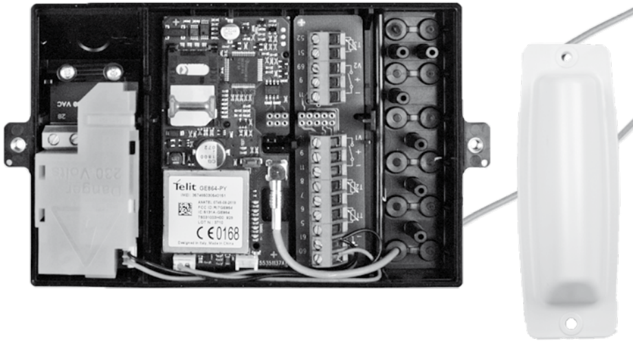
Fig. 4 – MULTICAL® 602
